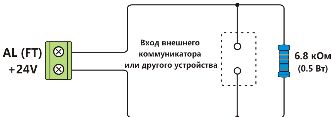
Рисунок 9 - Подключение выходов AL и FT
