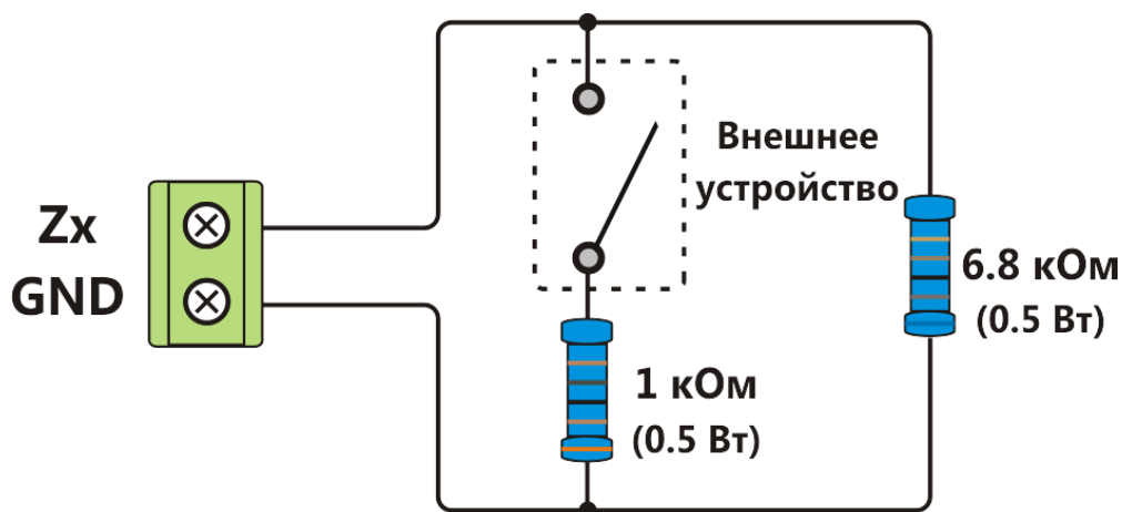
Рисунок 7 - Подключение универсального входа (под «x» следует понимать номер зоны)
