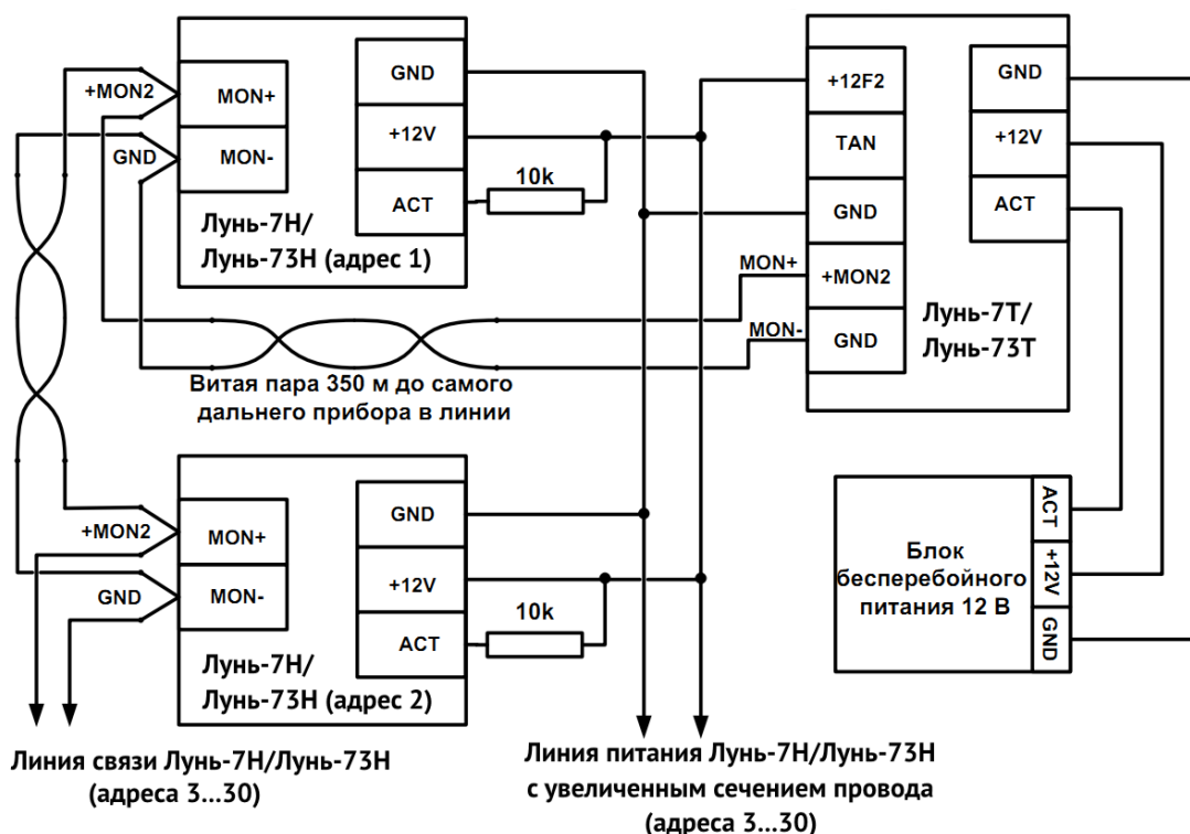
Рисунок 12. Схема подключения нескольких МР к базовому ППК
