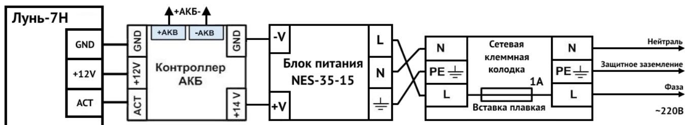
Рисунок 7. Подключение электропитания «Лунь-7Н»
