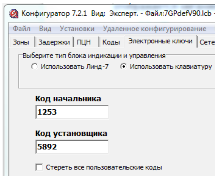
Рисунок 3. Ввод паролей
