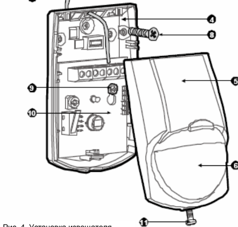
Рис. 4. Установка извещателя
