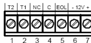
Рис. 6. Клеммная колодка
