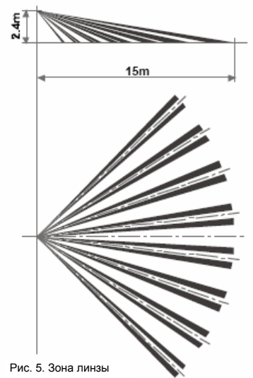
Рис. 5. Зона линзы
