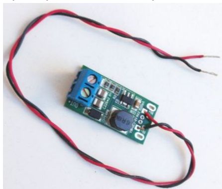
Рисунок 14. Адаптер DC-DC-5V-12V
