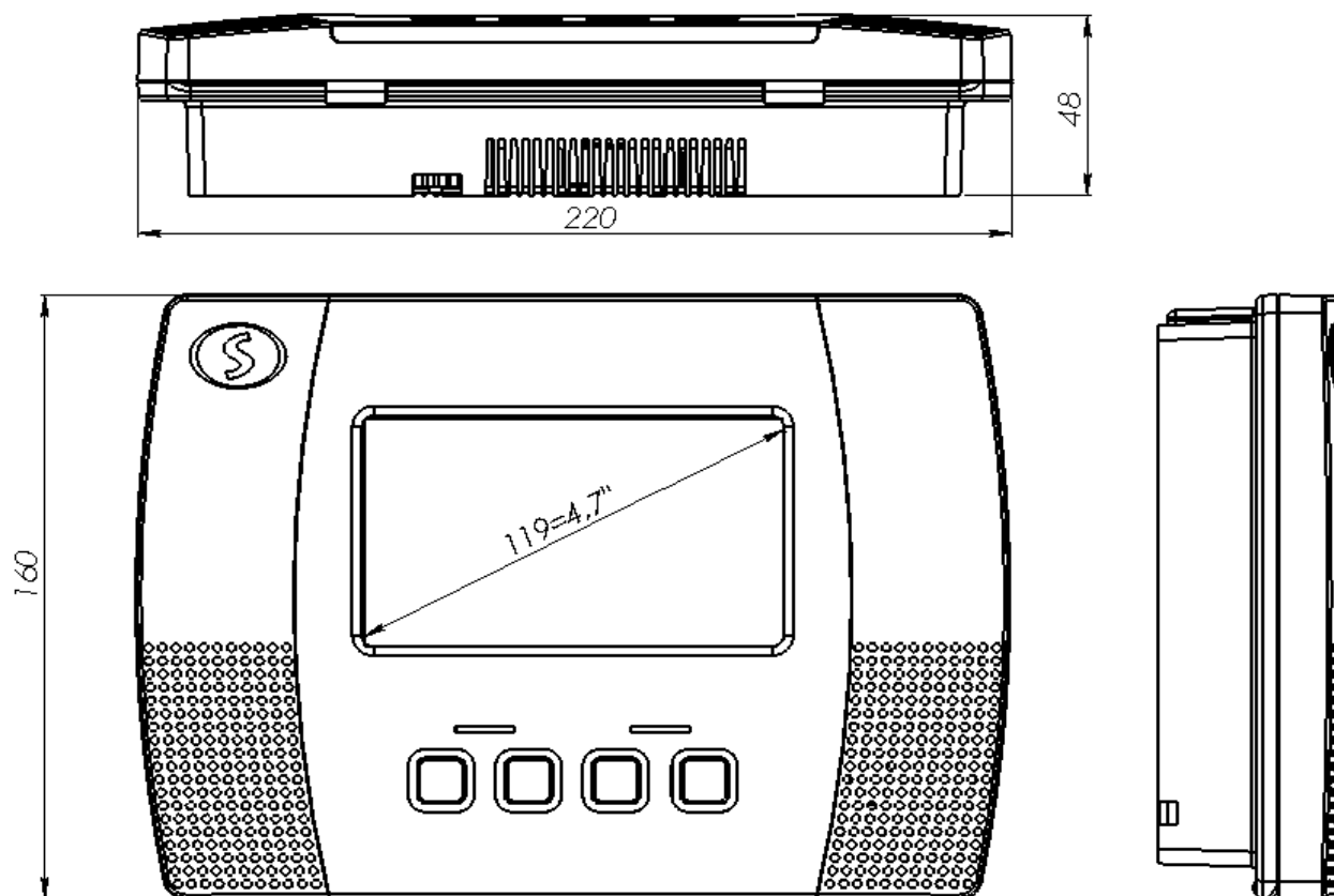
Рисунок 1. Внешний вид и габаритные размеры ППКОП
