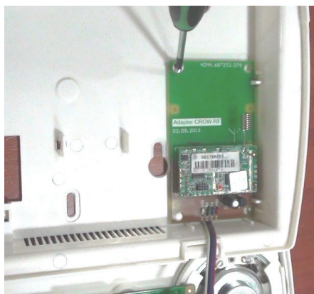
Рисунок 8. Установка адаптера «Crow-RF» в корпус
