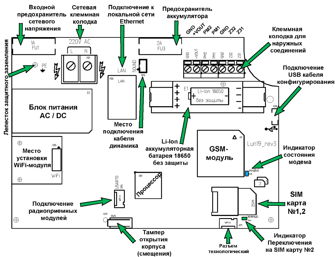
Рисунок 3. Схема расположения основных элементов на плате ППКОП
