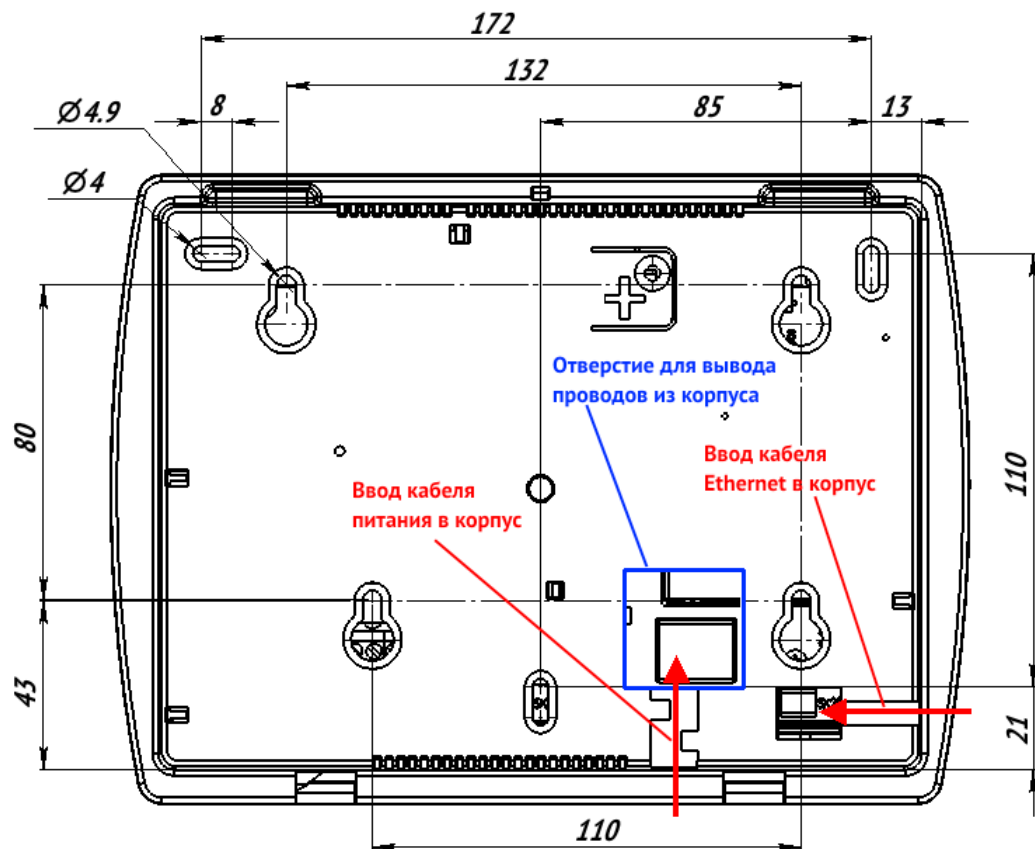
Рисунок 2. Установочные размеры корпуса ППКОП (вид со стороны установки)
