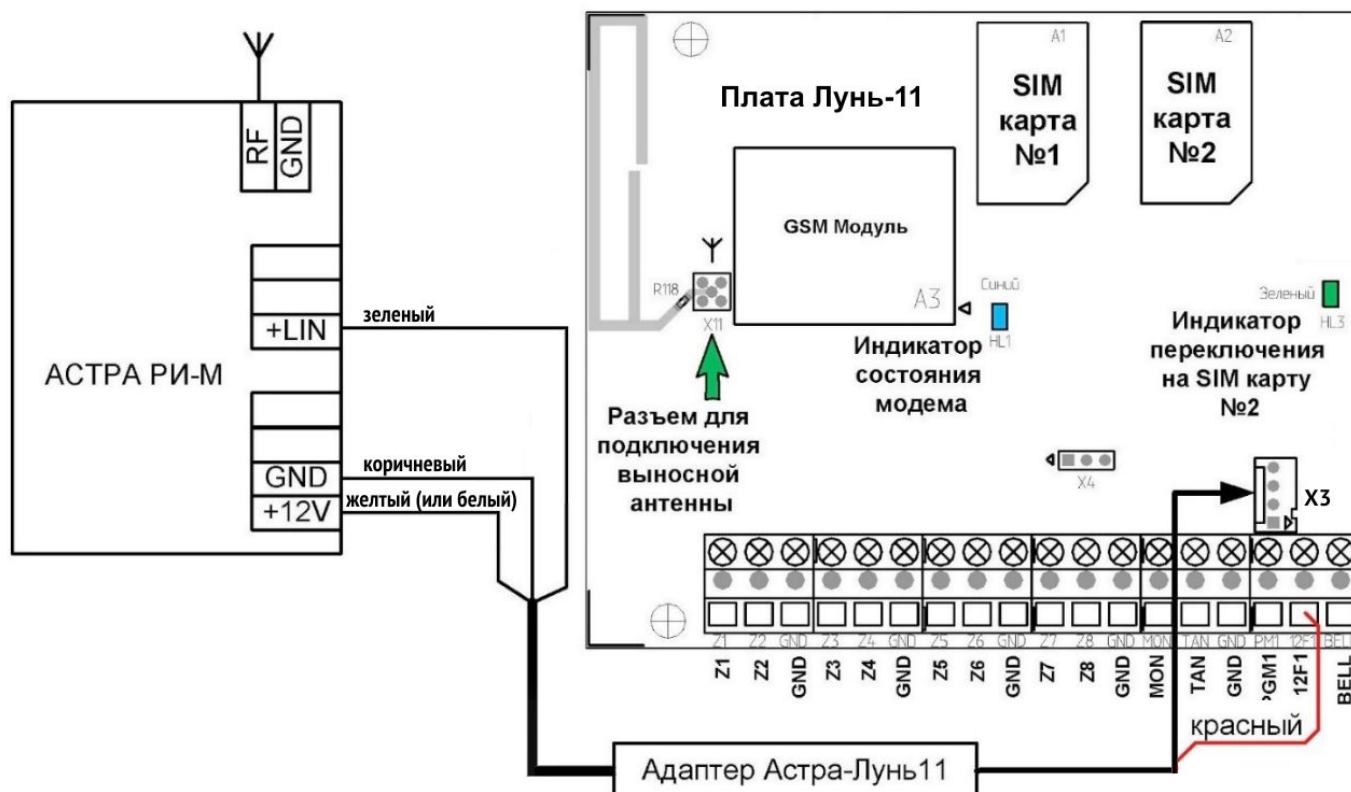
Рисунок 43. Схема подключения РПУ «Астра РИ-М»
