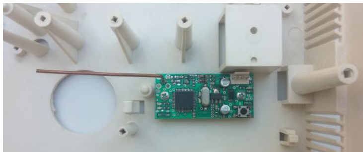
Рисунок 28. Радиоприемник Ajax «RR-108» в корпусе прибора
