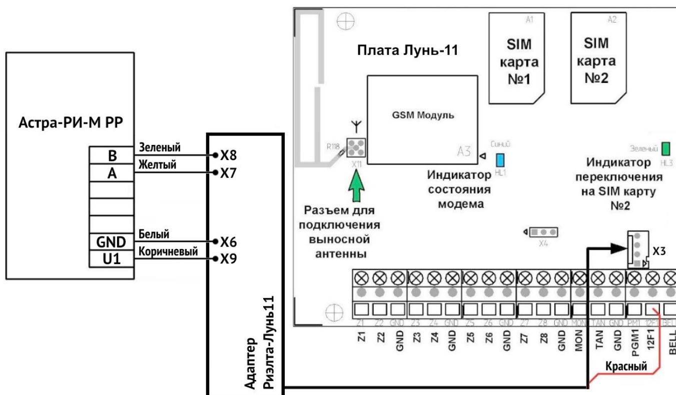
Рисунок 44. Схема подключения РПУ «Астра РИ-М РР»
