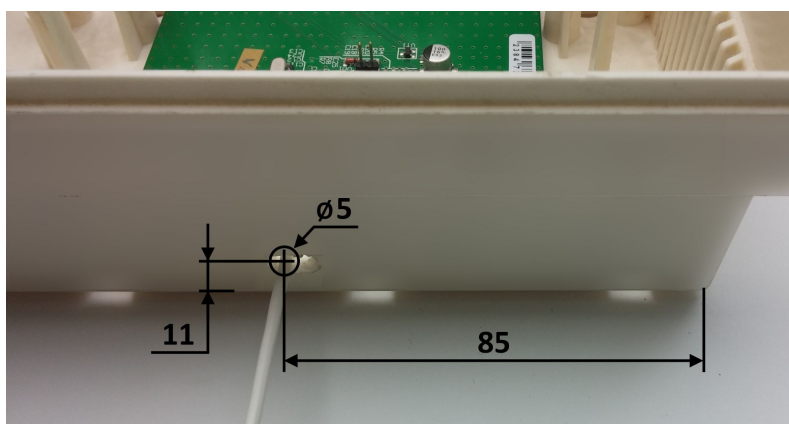
Рисунок 21. Отверстие в корпусе для антенны радиоприемника «P433» rev.4
