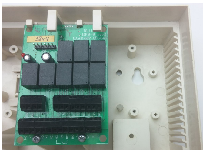
Рисунок 18. Модуль «МРВ-8М» в корпусе прибора
