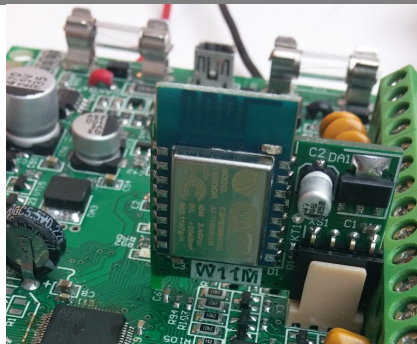
Рисунок 35. Установка модуля «W11M» в X3
