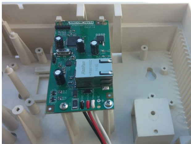
Рисунок 31. Коммуникатор «LanCom» rev.14 в корпусе прибора
