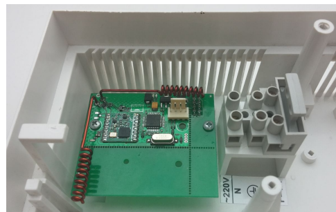
Рисунок 29. Радиоприемник Ajax «uartBridge» в корпусе прибора
