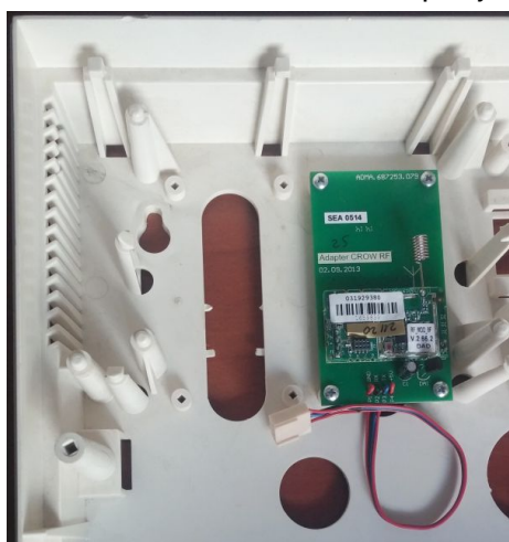
Рисунок 25. Адаптер «Crow – Лунь-11» в корпусе прибора
