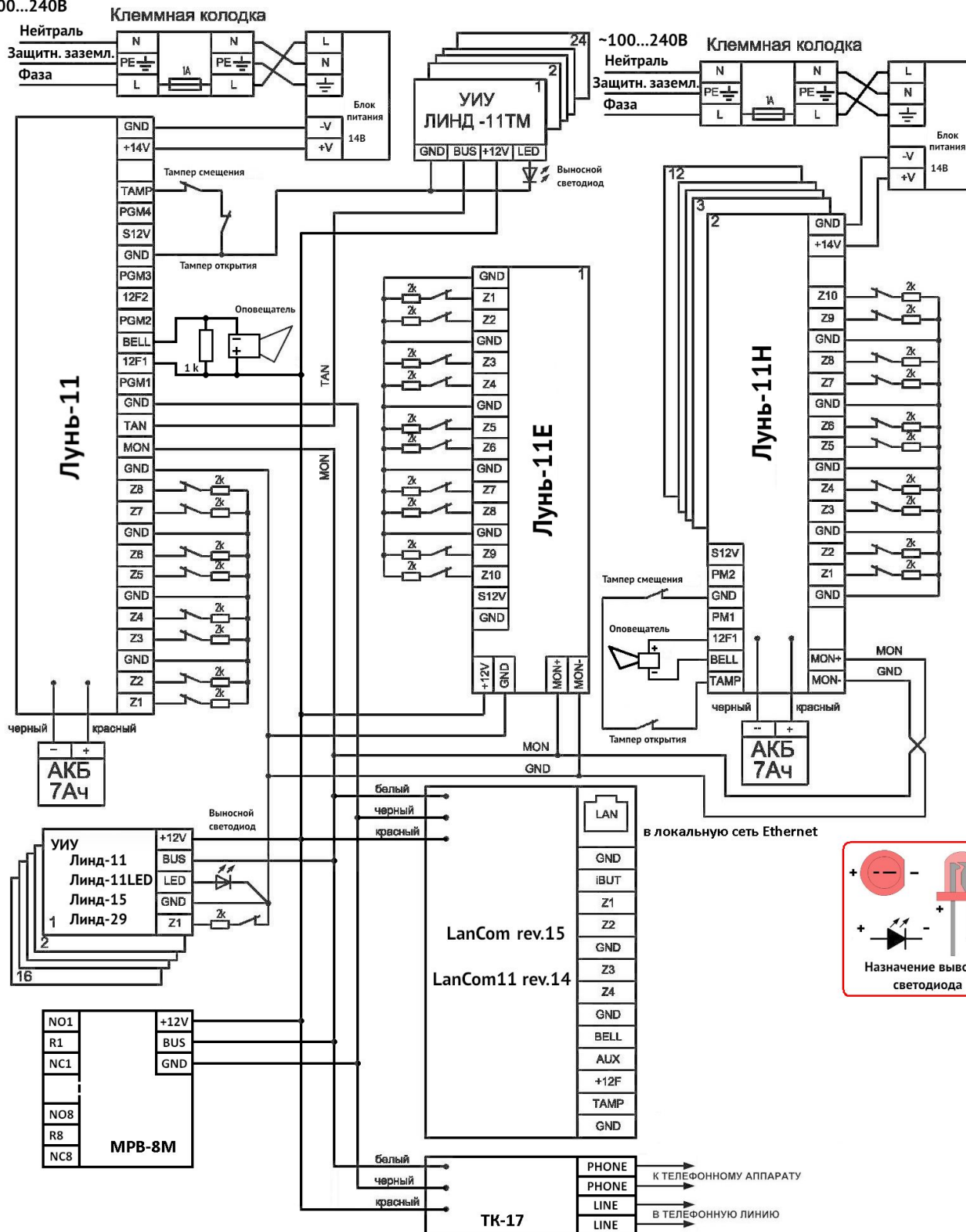
Рисунок 41. Схема подключения сетевых устройств
