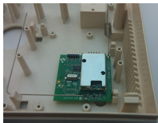
Рисунок 22. Радиоприемник «MCR-300» Visonic в корпусе прибора
