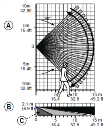
A. HORIZONTALE ANSICHT B. VERTIKALE ANSICHT C. PG8904P: 2-4m (6.5 – 13ft)
