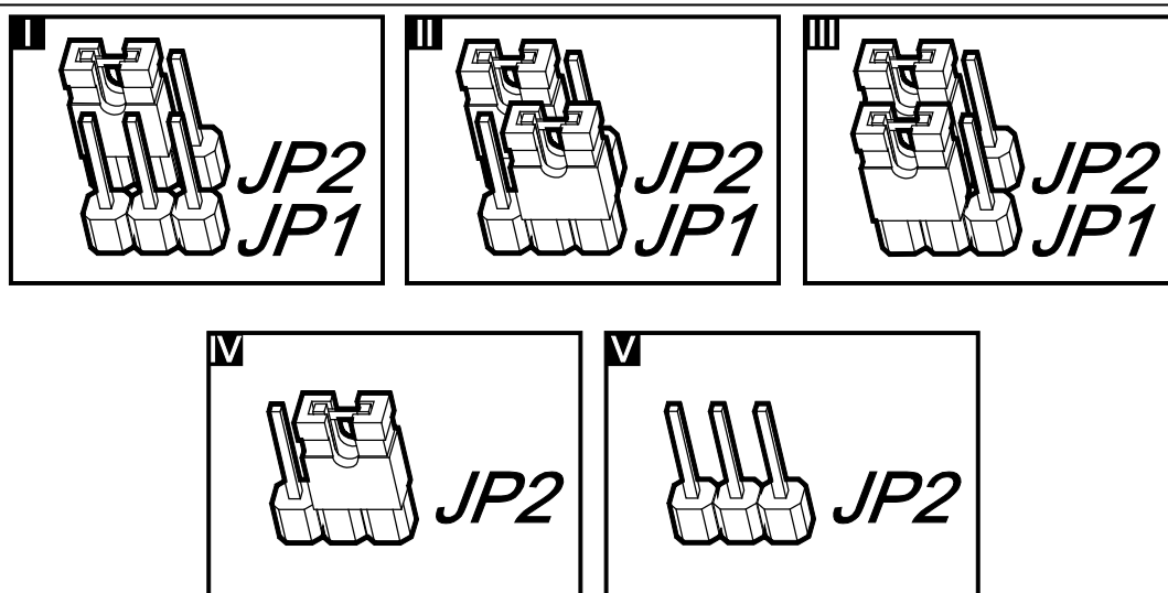
Рис. 3. Способ установки перемычек для выбора типа оптической сигнализации.
