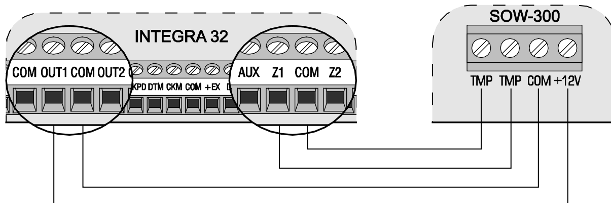
Рис. 5. . Способ подключения SOW-300 к ПКП – сигнализация должна активироваться подачей напряжения +12 В (активацией силового выхода OUT1 с положительной поляризацией). Зону Z1 следует запрограммировать как 24 ч саботажная.
