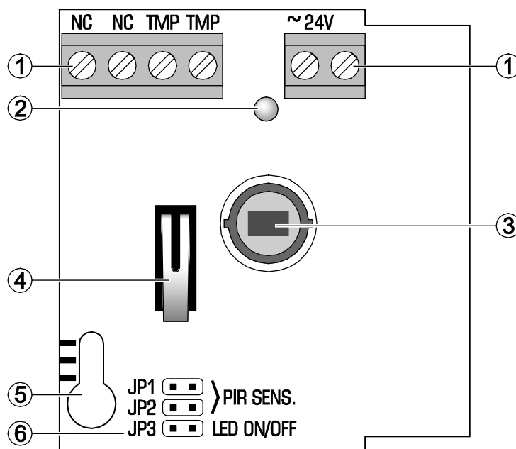
Рис.1. Вид платы электроники извещателя.
